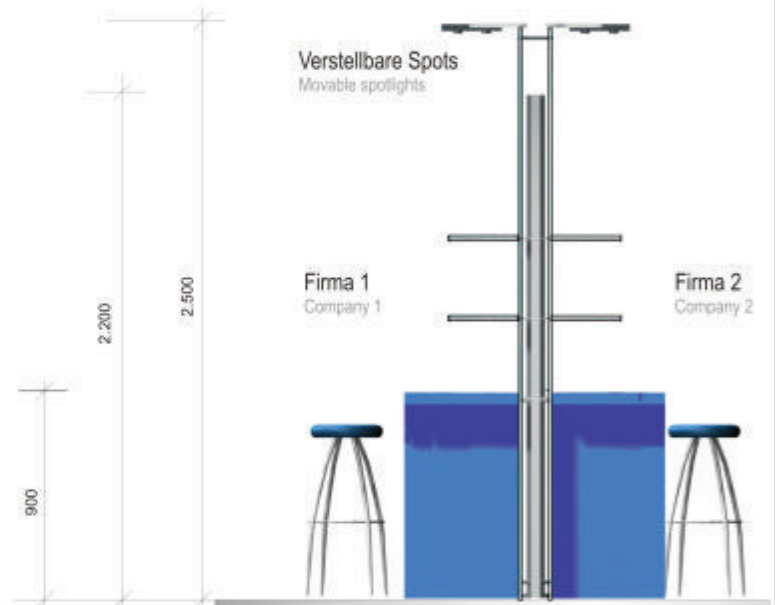
Schnitt Section
