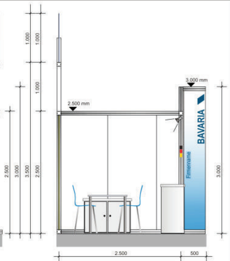
Schnitt Section
