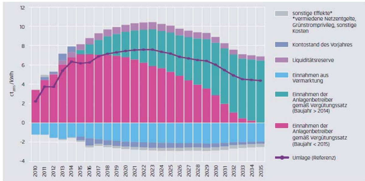
Abbildung 23: Mögliche Entwicklung der EEG-Umlage bis 2035
